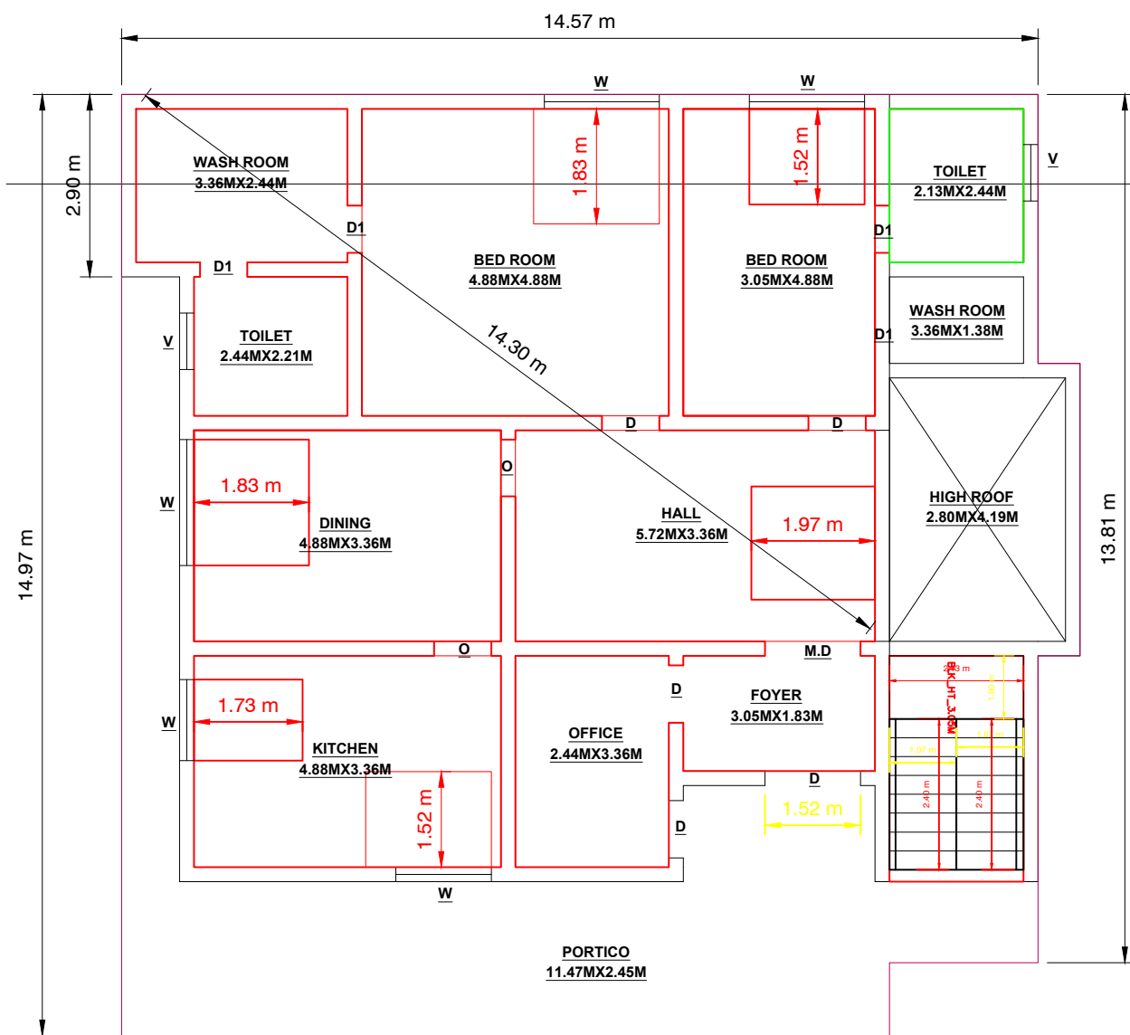
G.F PLAN
