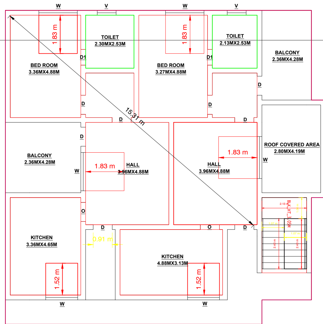
F.F PLAN
