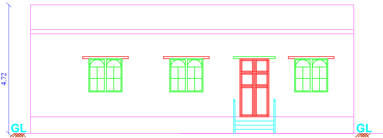
ELEVATION
