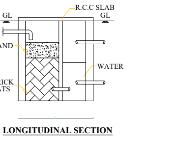
LONGITUDINAL SECTION
