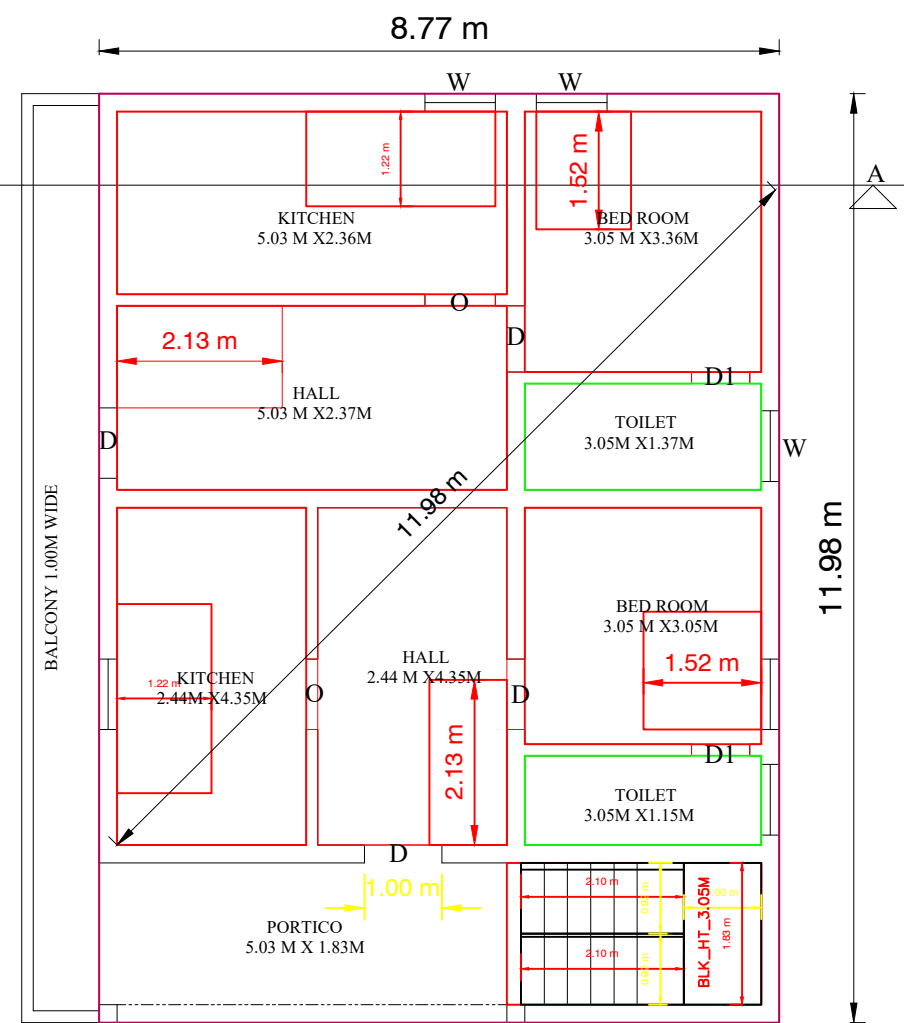
PRO- F.F PLAN
