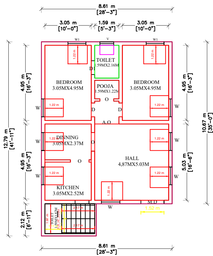
PLAN SCALE ( 1 : 100 )
