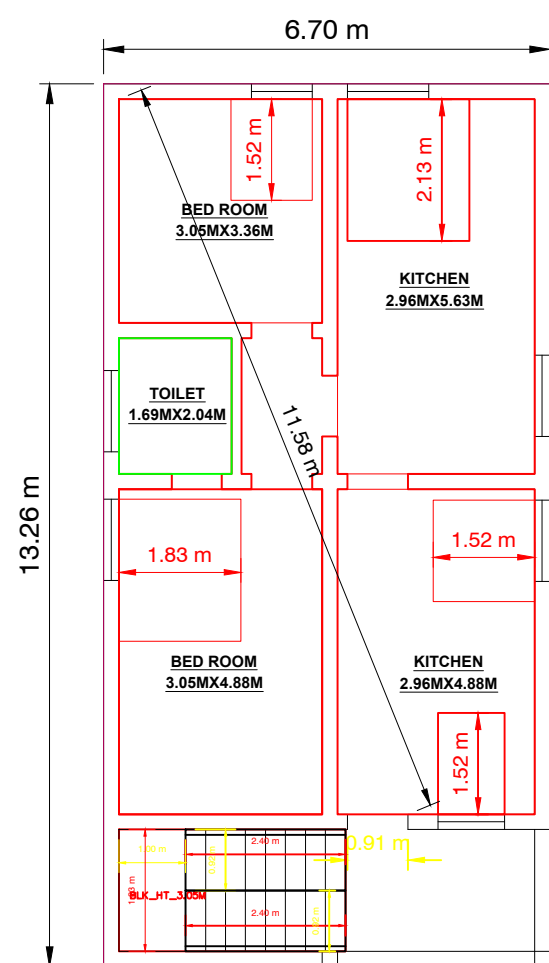
G.F PLAN
