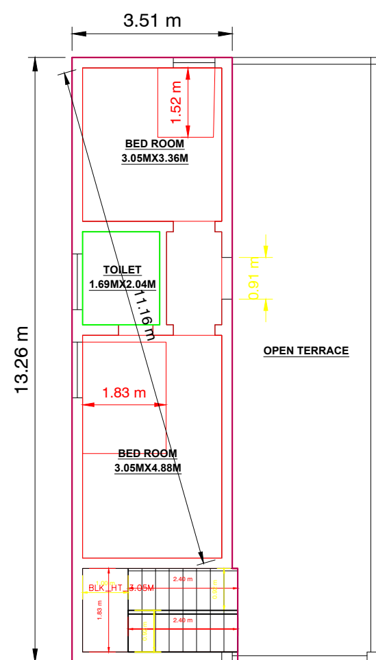
F.F PLAN
