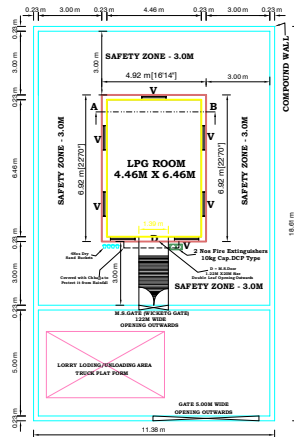
GODOWN - PLAN
