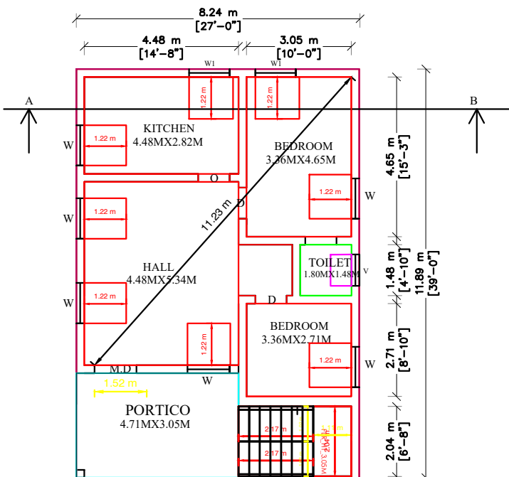
PLAN SCALE ( 1 : 100 )
