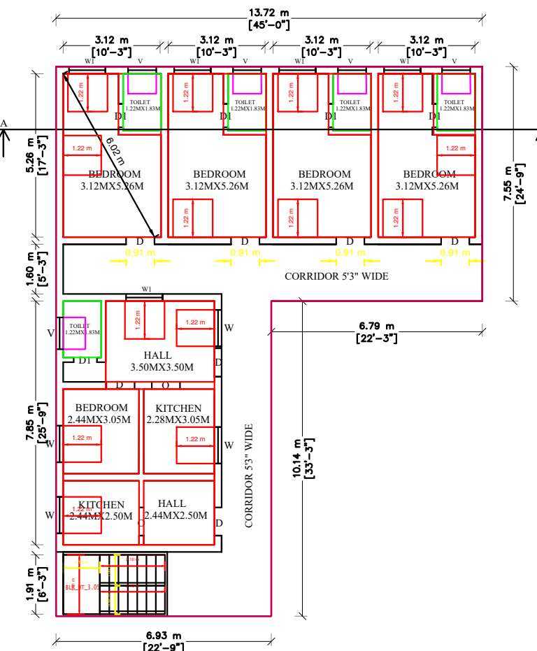
PLAN SCALE ( 1 : 100 )
