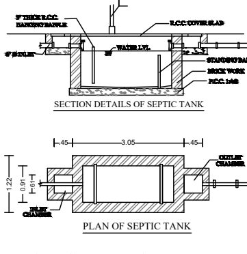
DETAILS OF SEPTIC TANK (N.T.S.)
