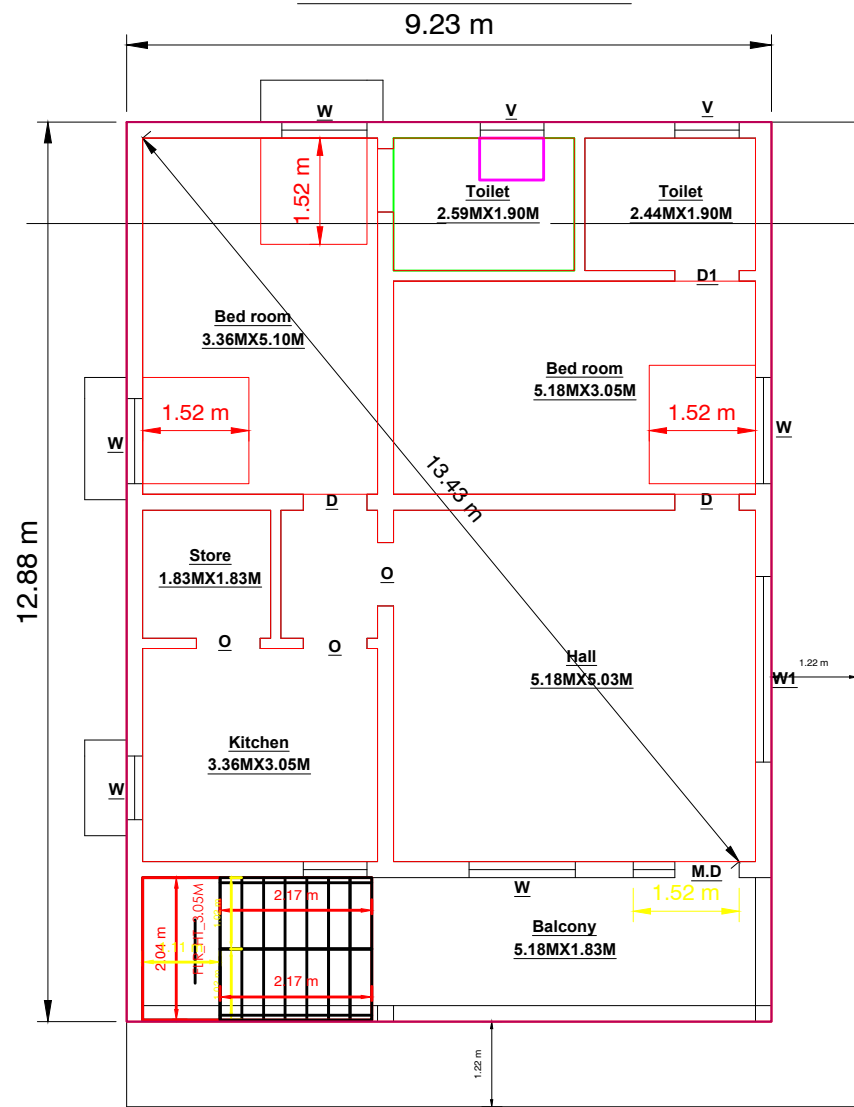
F.F PLAN
