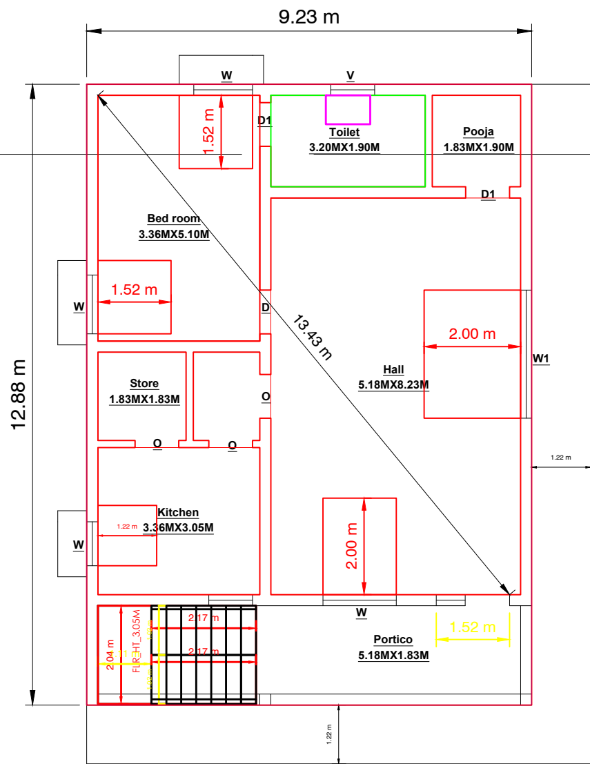
G.F PLAN
