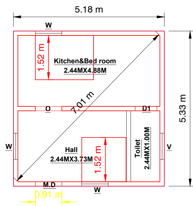
G.F PLAN
