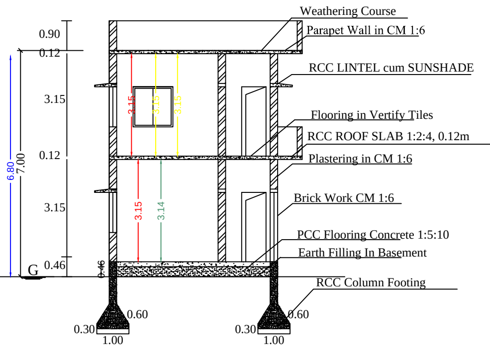
SECTION - AB
