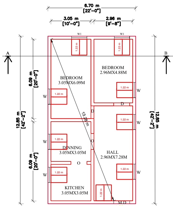
PLAN SCALE ( 1 : 100 )
