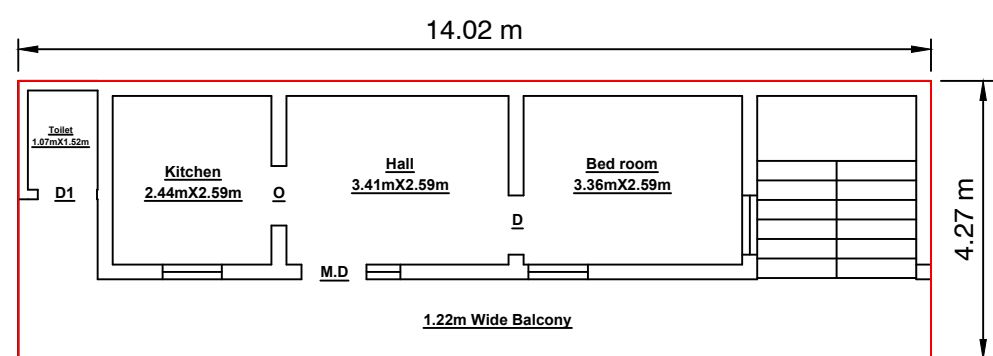
F.F PLAN
