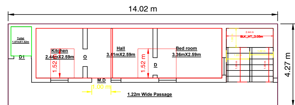
G.F PLAN
