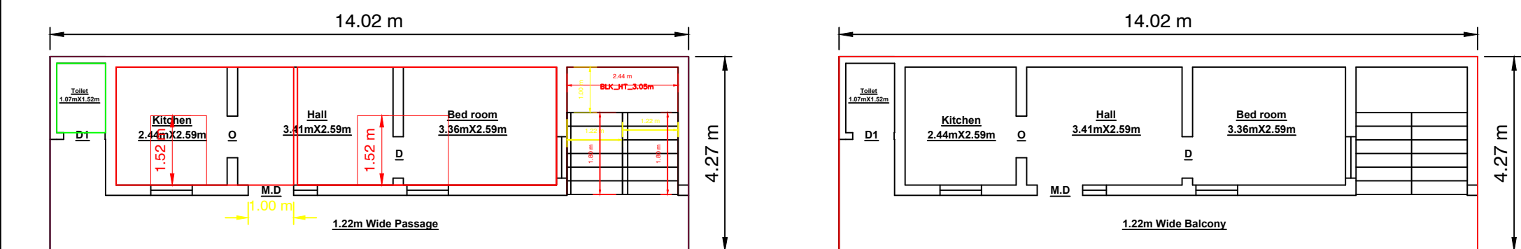
G.F PLAN
