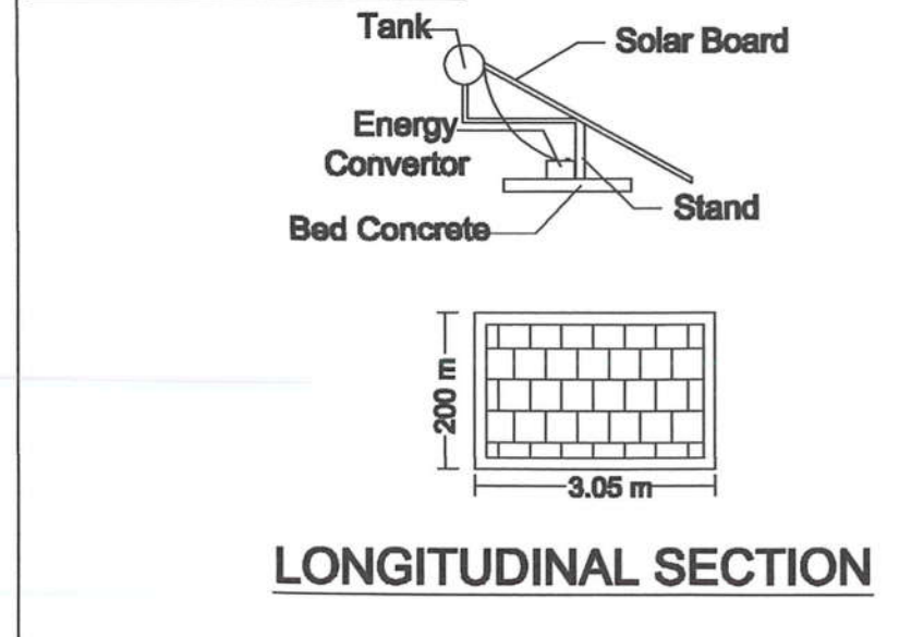
SOLAR PANEL N.T.S
