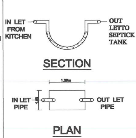
'U' TRAP
