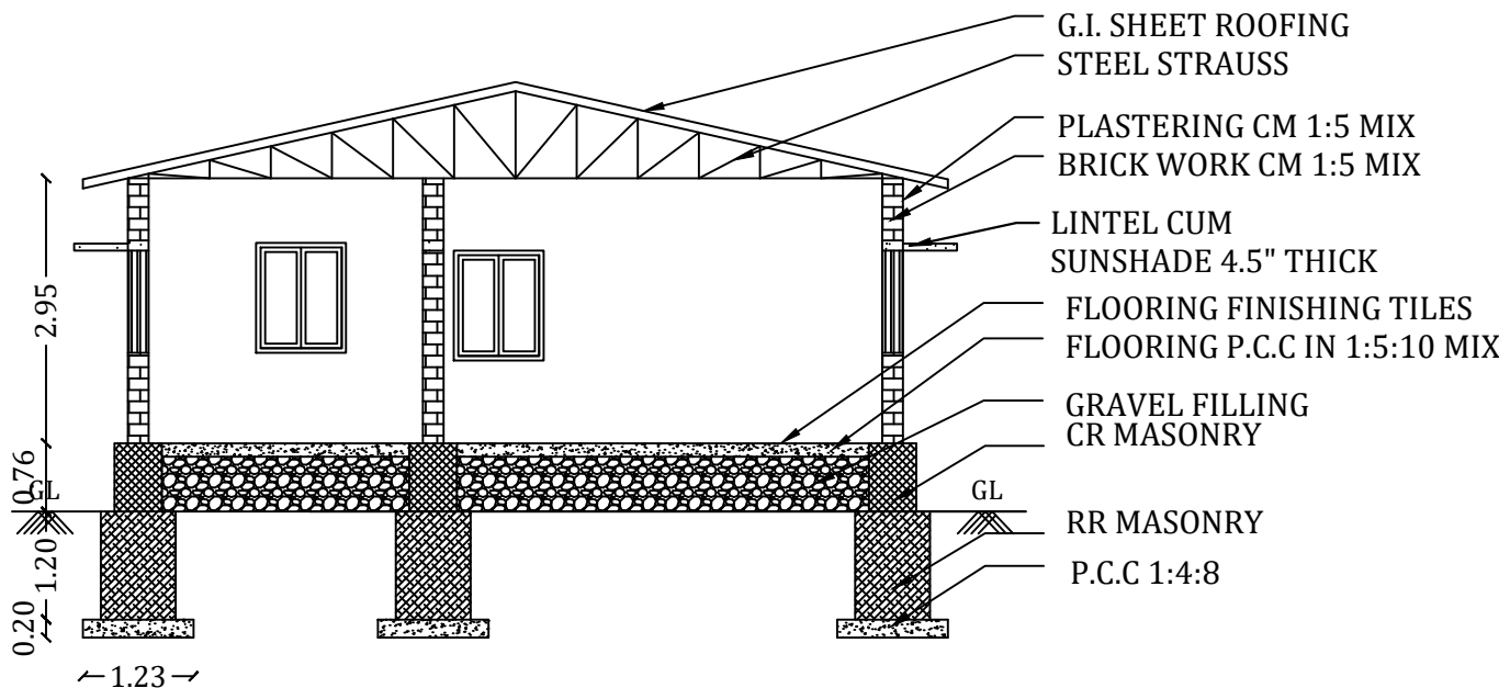
SECTION A-B
