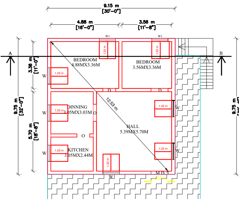
PLAN SCALE ( 1 : 100 )
