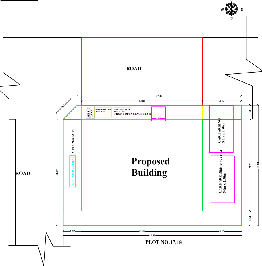
SITE PLAN 1:100 SCALE
