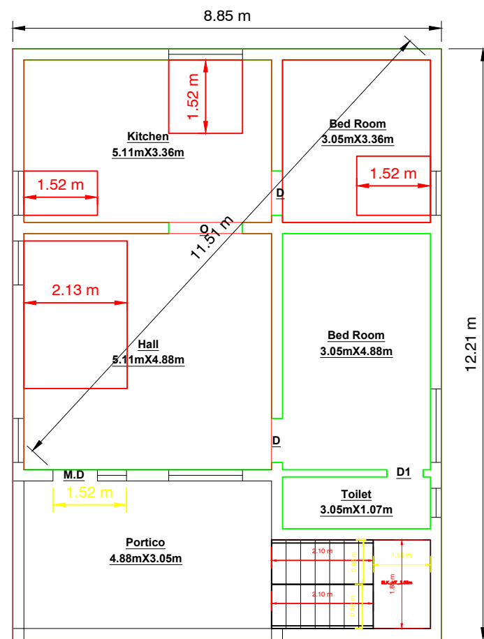
G.F PLAN
