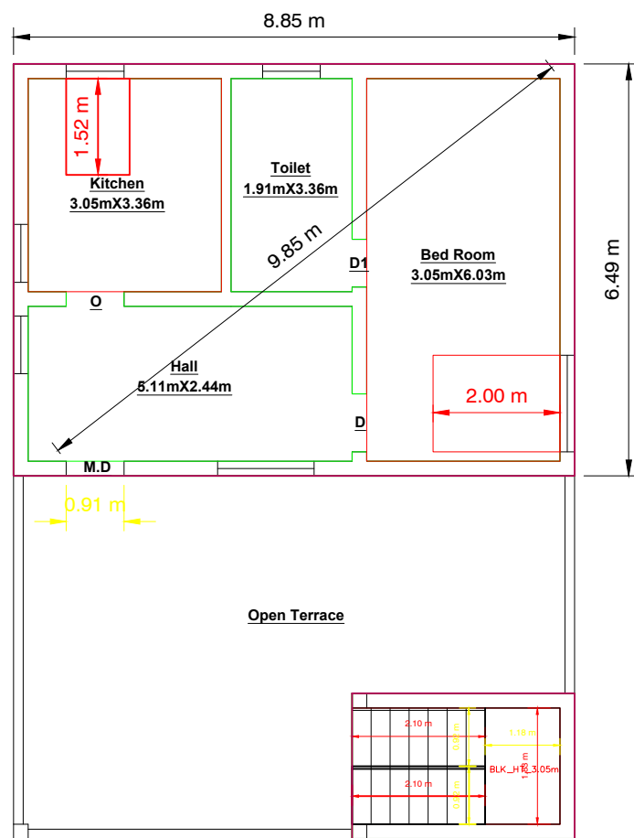
F.F PLAN
