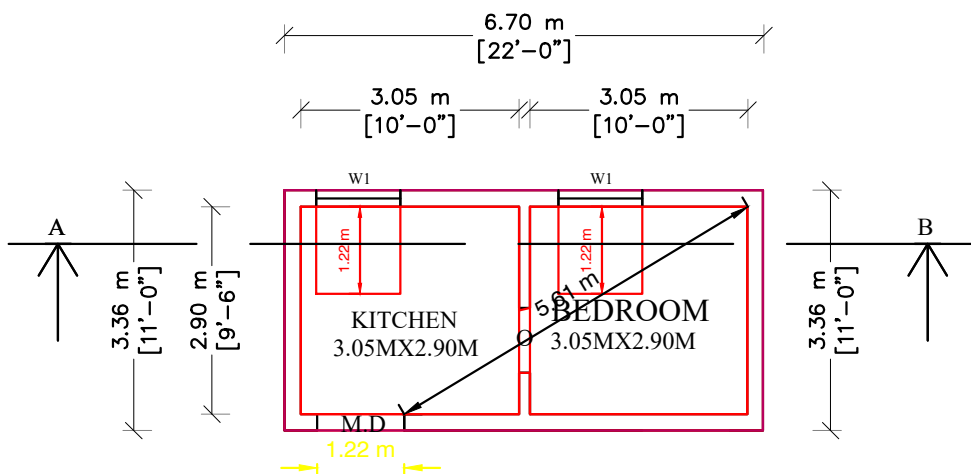
PLAN SCALE ( 1 : 100 )
