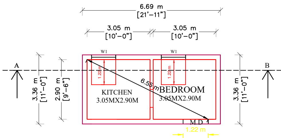
PLAN SCALE ( 1 : 100 )
