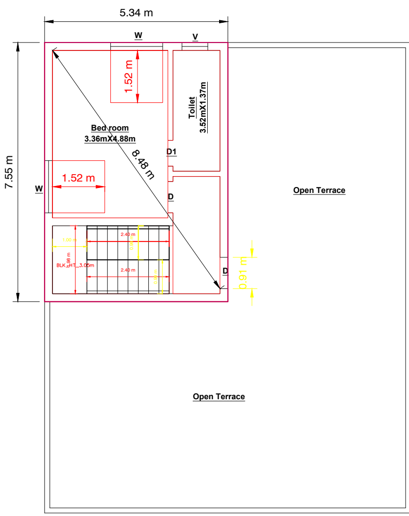
F.F PLAN
