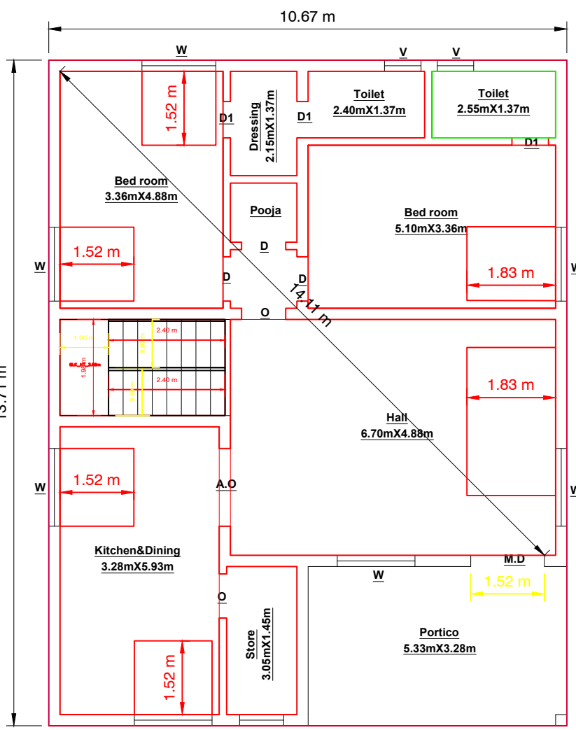
G.F PLAN
