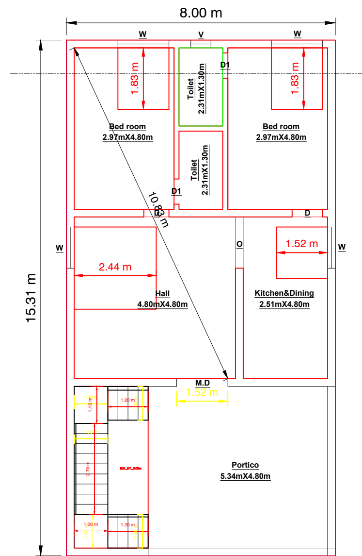
G.F PLAN
