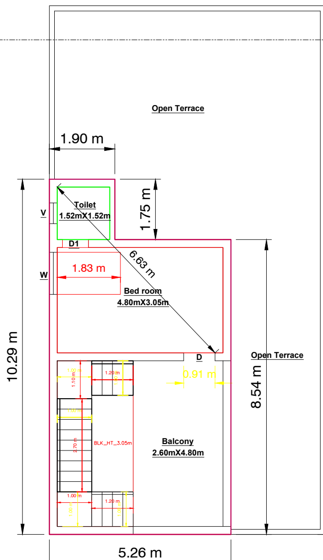
F.F PLAN
