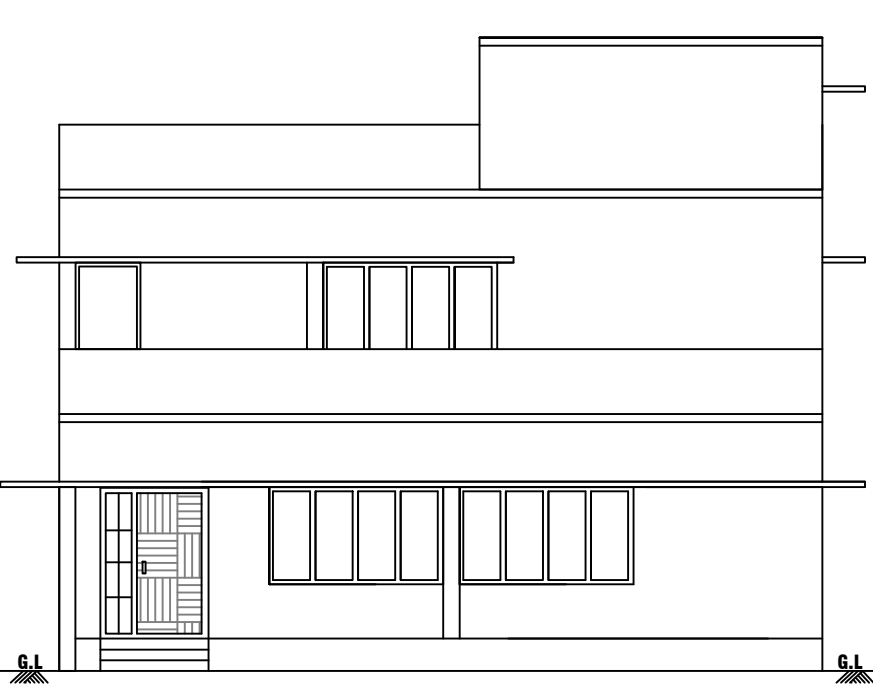
ELEVATION
