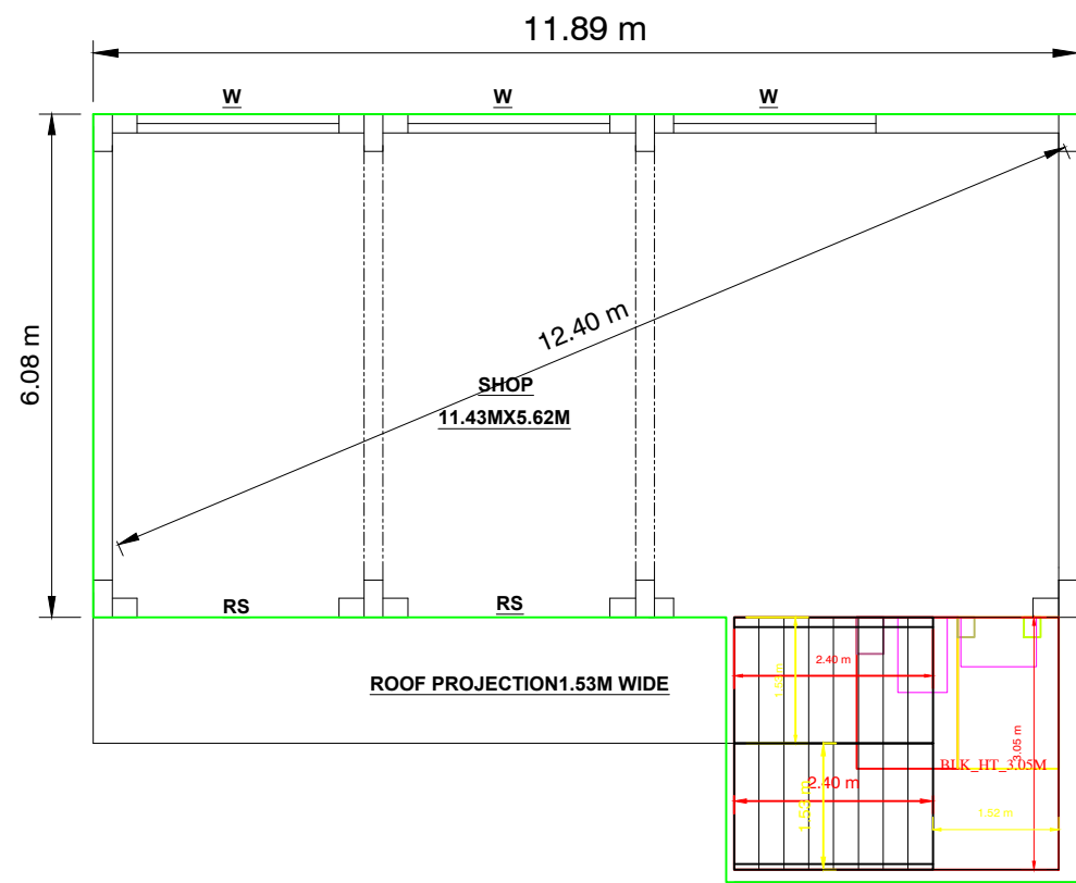
EXI- G.F PLAN
