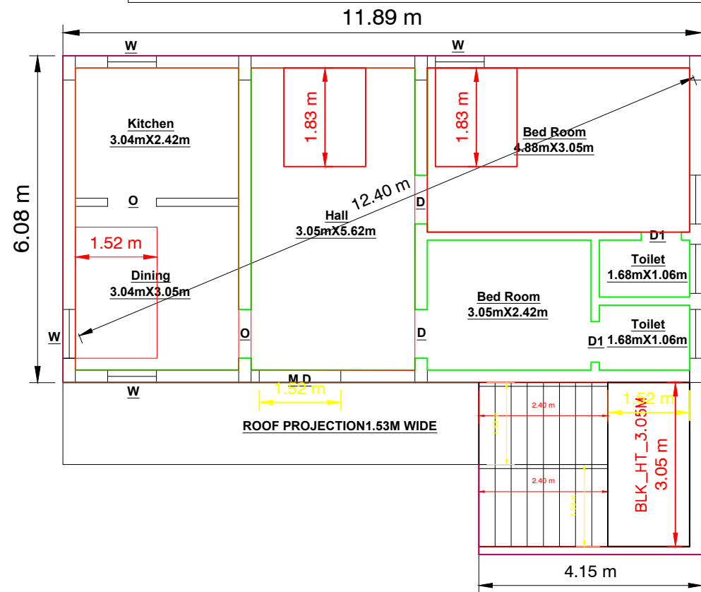
PRO-S.F PLAN
