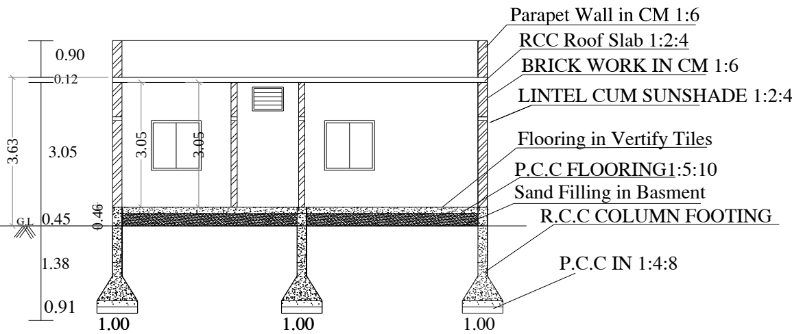
SECTION - AB
