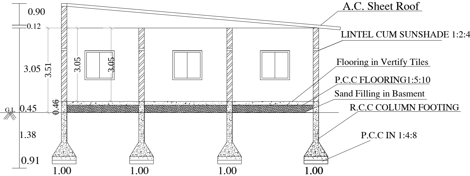
SECTION - AB
