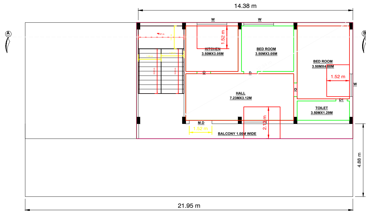
PRO-S.F PLAN
