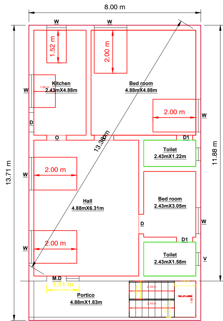
G.F PLAN
