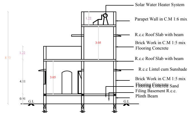
SECTION A-B
