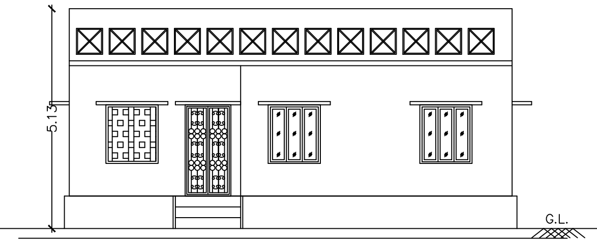
ELEVATION
