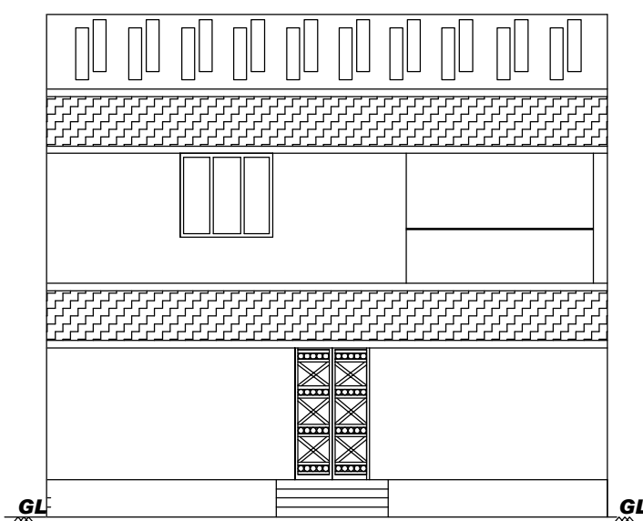
ELEVATION
