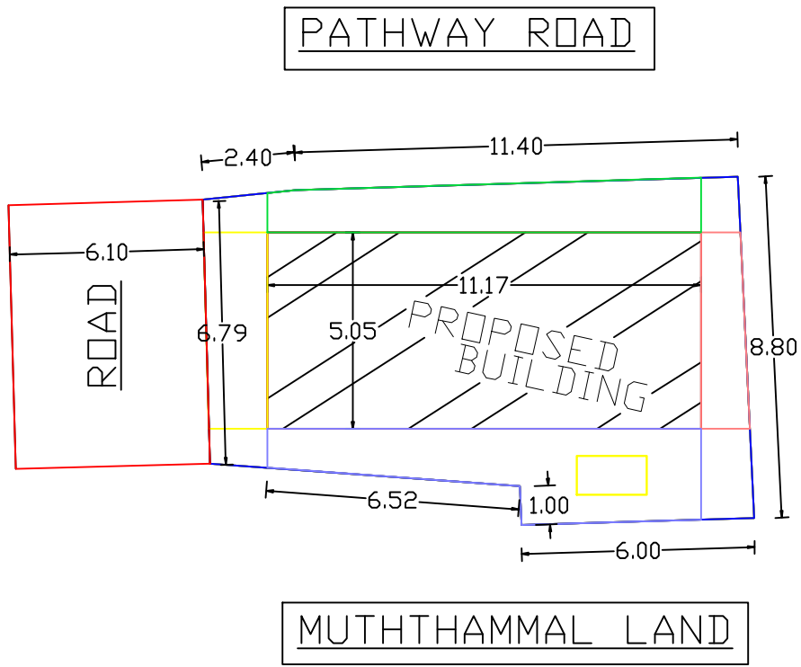
SITE PLAN 1:100 SCALE
