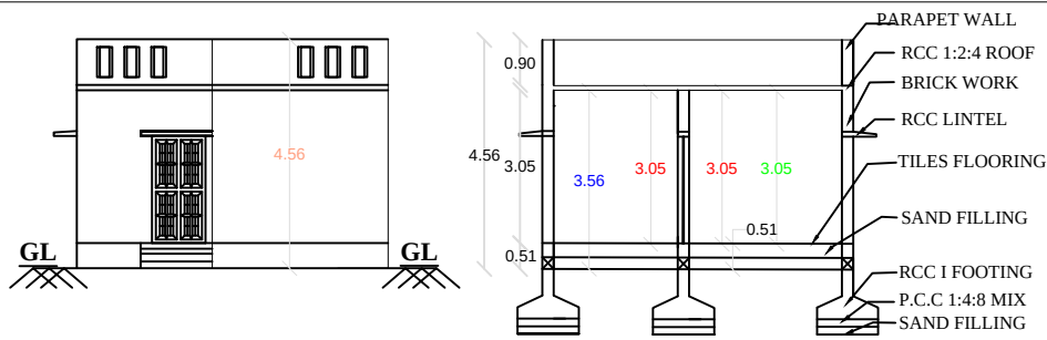
ELEVATION
