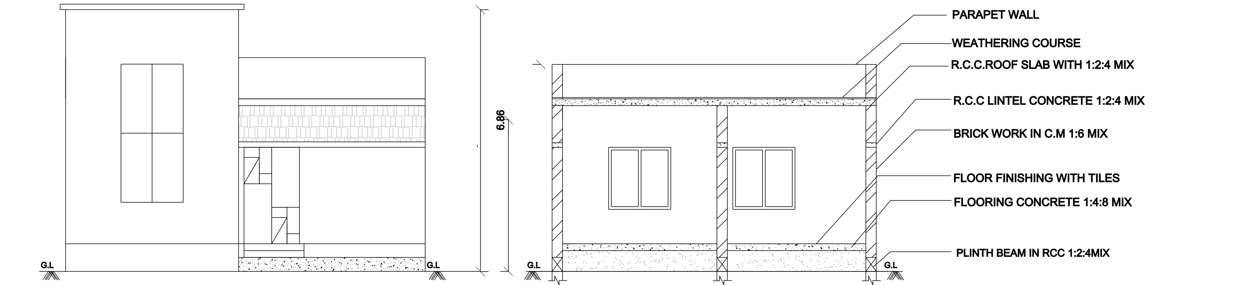
ELEVATION
