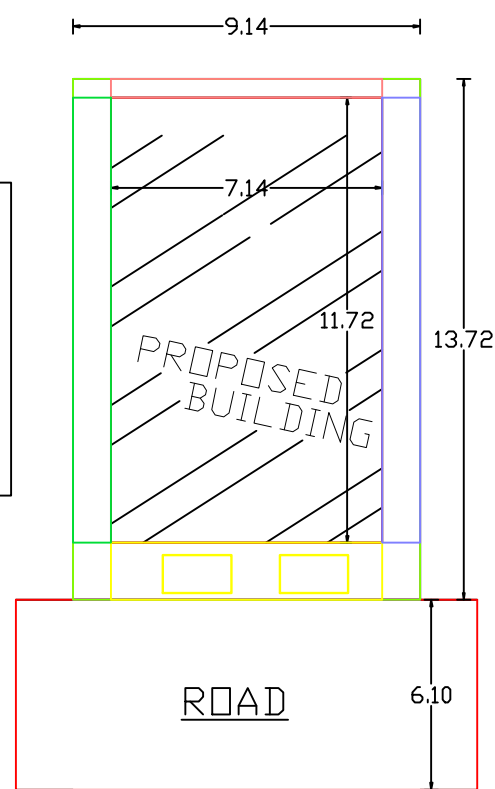
SITE PLAN 1:100 SCALE
