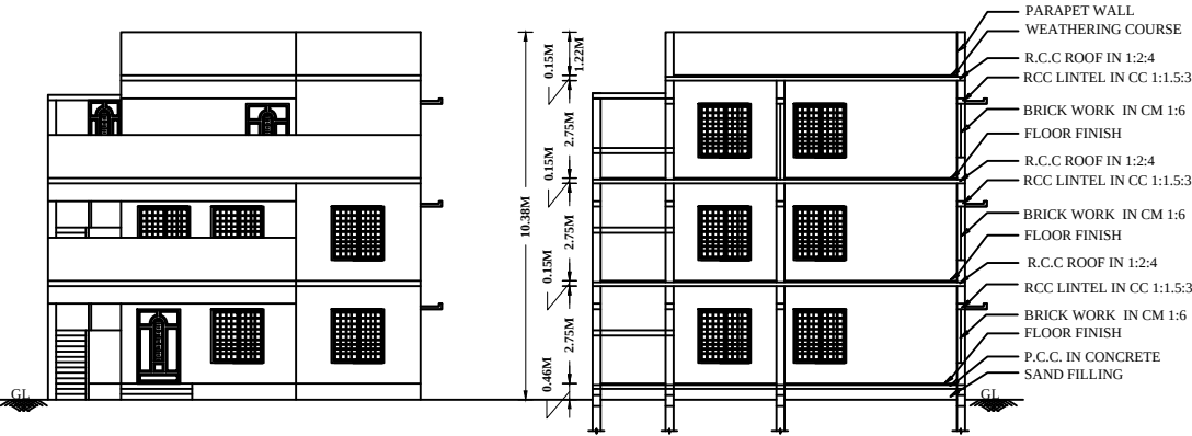
ELEVATION
