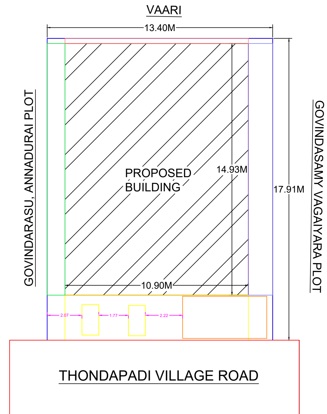
SITE PLAN 1:100 SCALE
