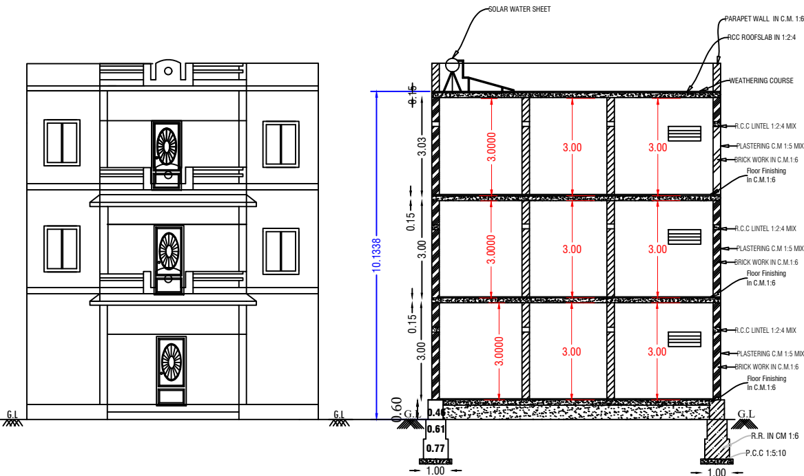
ELEVATION
