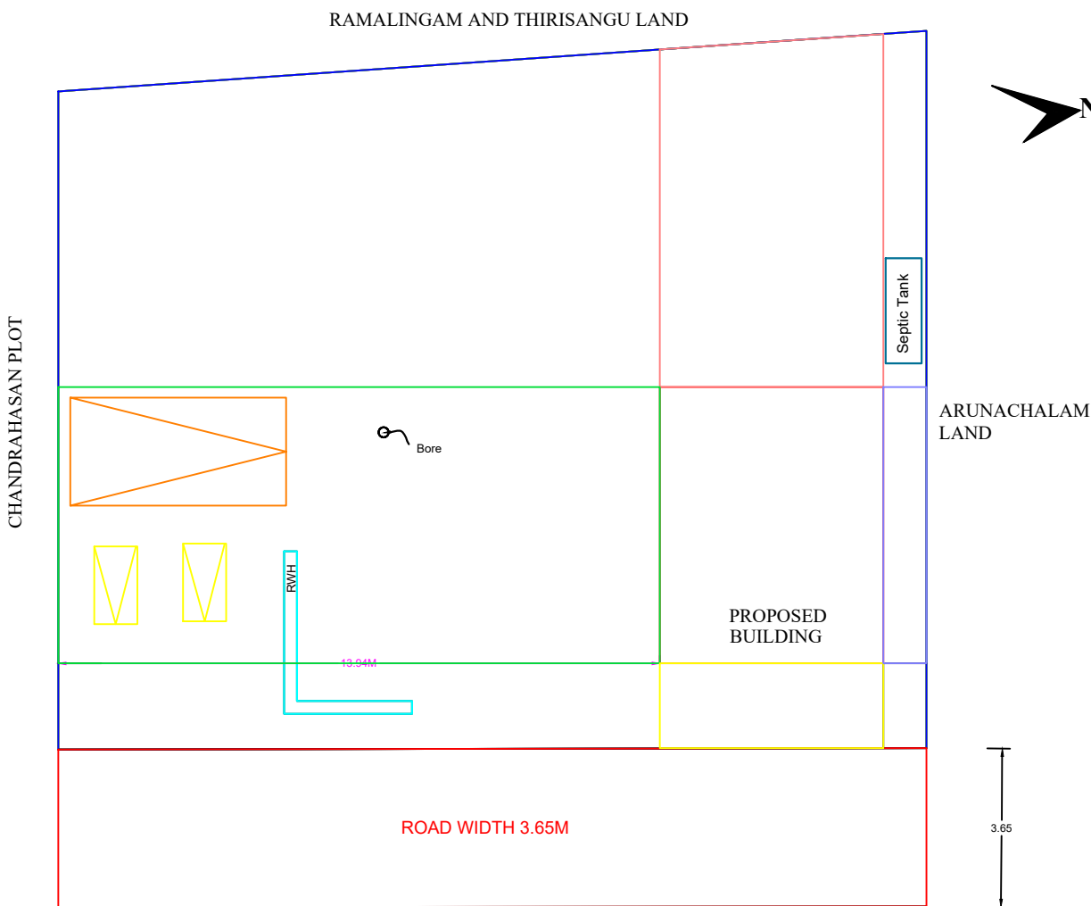
SITE PLAN 1:100 SCALE
