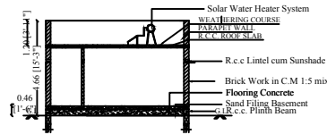
SECTION A-B
