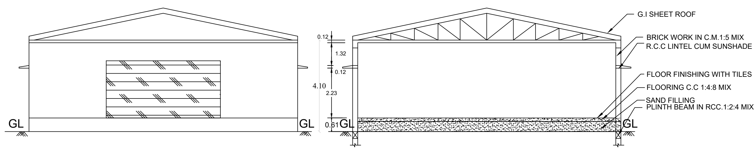
ELEVATION
