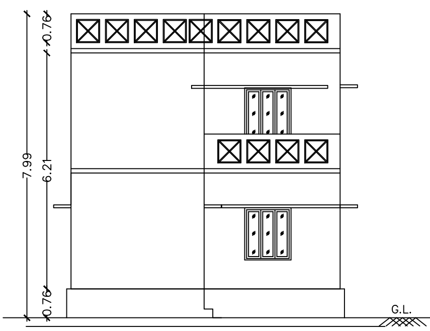
ELEVATION
