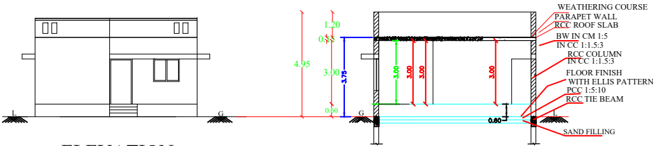
ELEVATION
