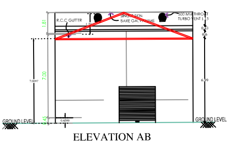
ELEVATION AB
