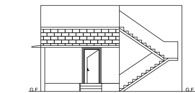
ELEVATION
