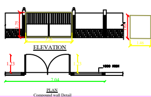
ELEVATION
