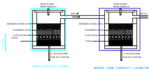
RWH_CAPACITY_L=1000
