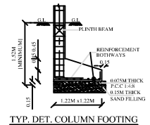
TYP. DET. COLUMN FOOTING
