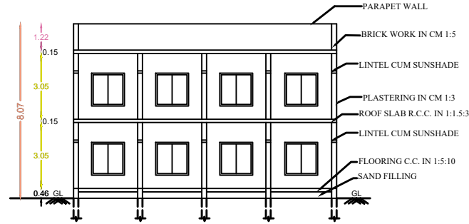
SECTION NO A-A
